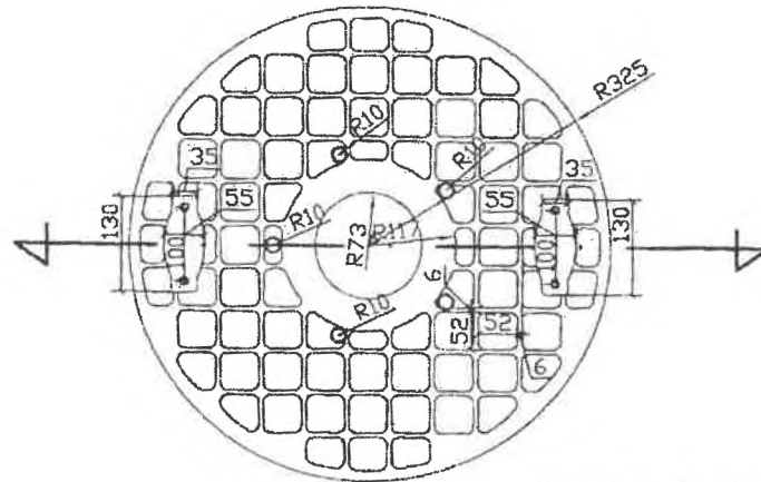
Изглед отгоре
