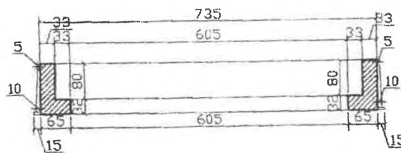
Разрез
