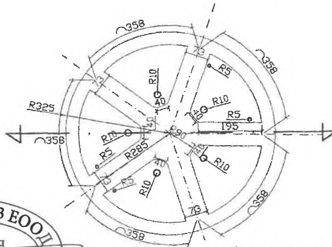
Изглед отдолу
