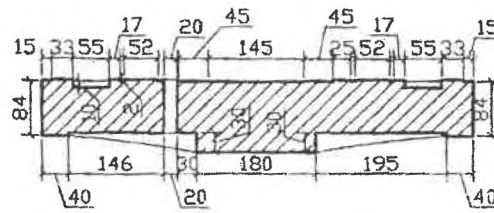
Разрез
